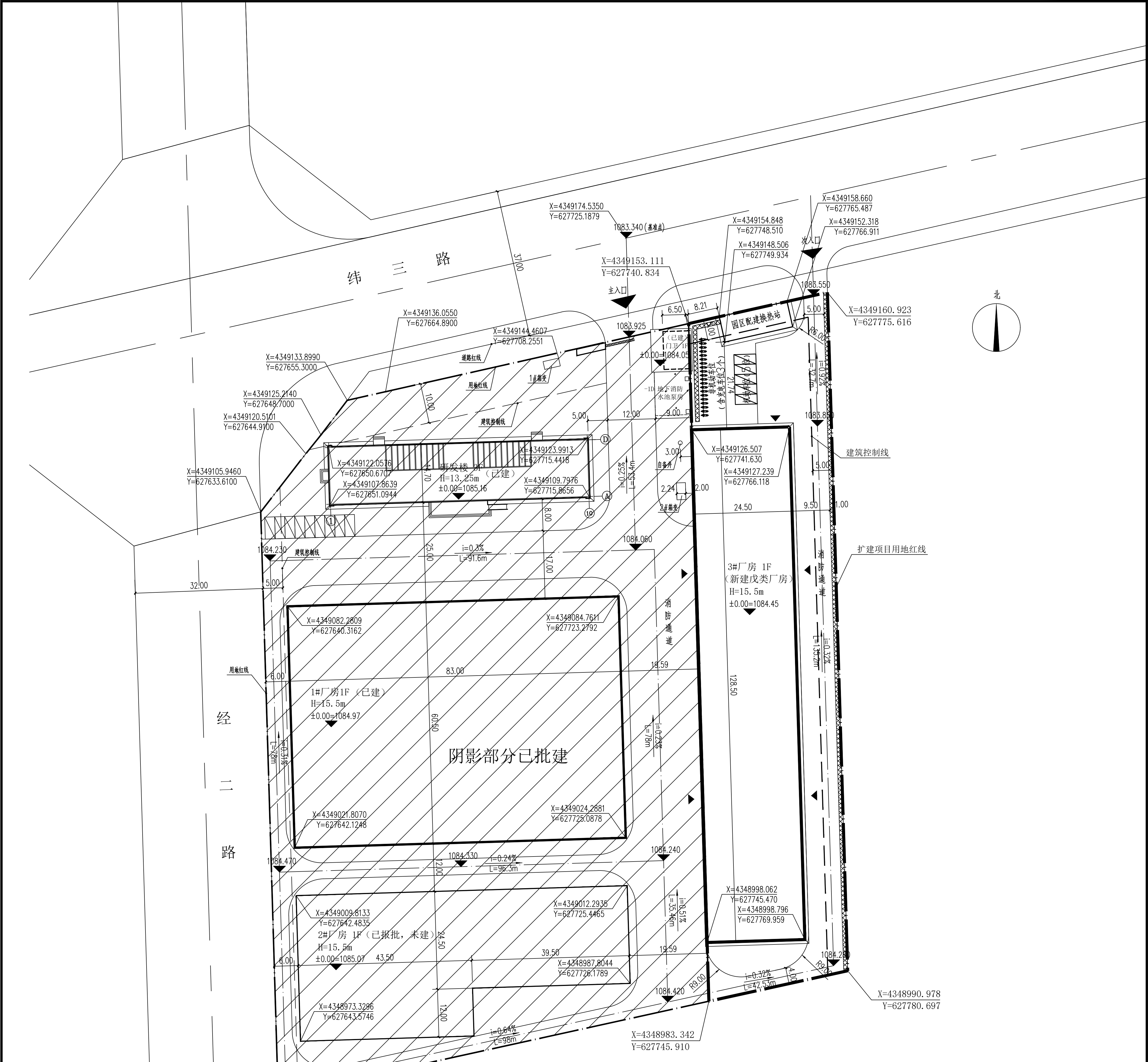
总平面图 1:500
